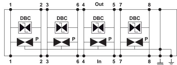
Příklad: zapojení MJ8-CAT5E
